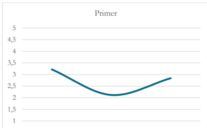
Slika 2: Primer grafa
